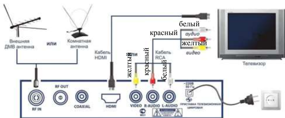
Рис. 6. Схема приема цифрового телевизионного сигнала
